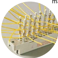
Fig. X-3: Modified wrap
